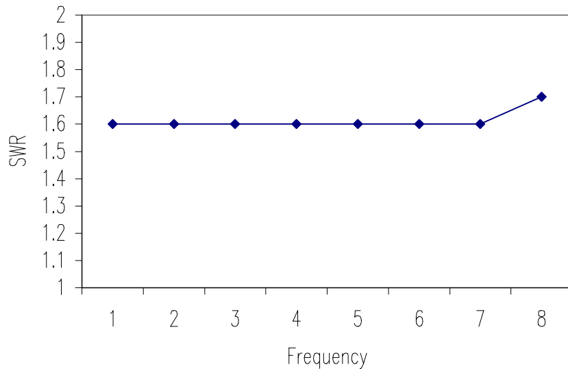
SWR 20m
